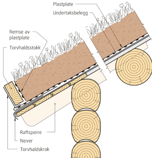
Fig. 22 Eksempel på oppbygning av torvtak over oppvarmet bygning. Taket har tettesjikt av undertaksbelegg og plastplate.
